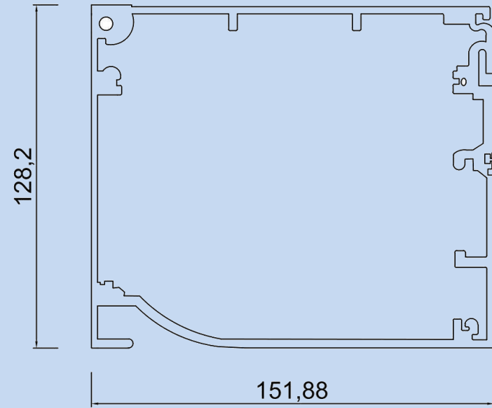
5)Κουτί μοτέρ Motor box profile
