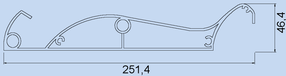
6)Προφίλ περσίδας Louvre profile
